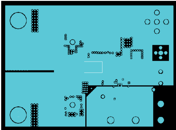
Fig. 10 - Inner Layer1
