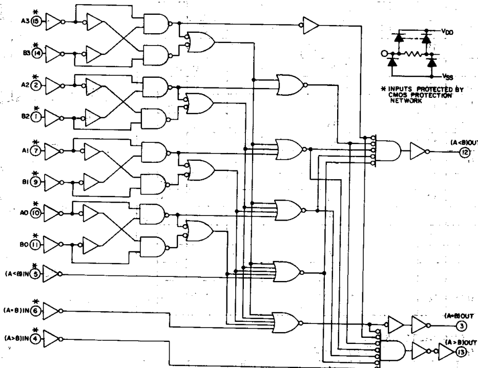
Fig. 4 - Logic diagram.
