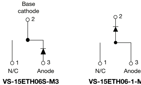
VS-15ETH06S-M3
